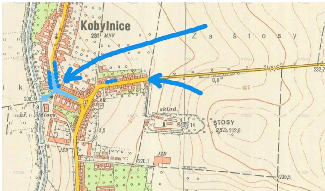
Na mapce (z roku 1952, ale obec se za tu dobu tolik nezměnila) je možné vidět, kudy se voda valila a které domy byly poškozeny.
